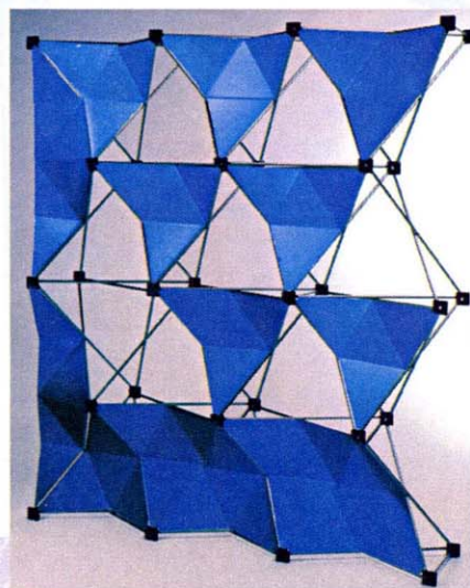
意匠的に三角パネルを一部はずした例
